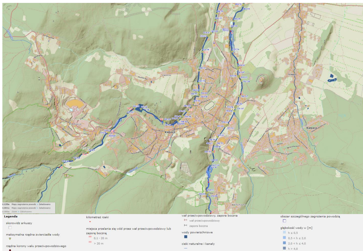
Rysunek 12 Mapy zagrożenia powodziowego dla gminy Karpacz z uwzględnieniem Q0,2%, Q1% oraz Q10%
