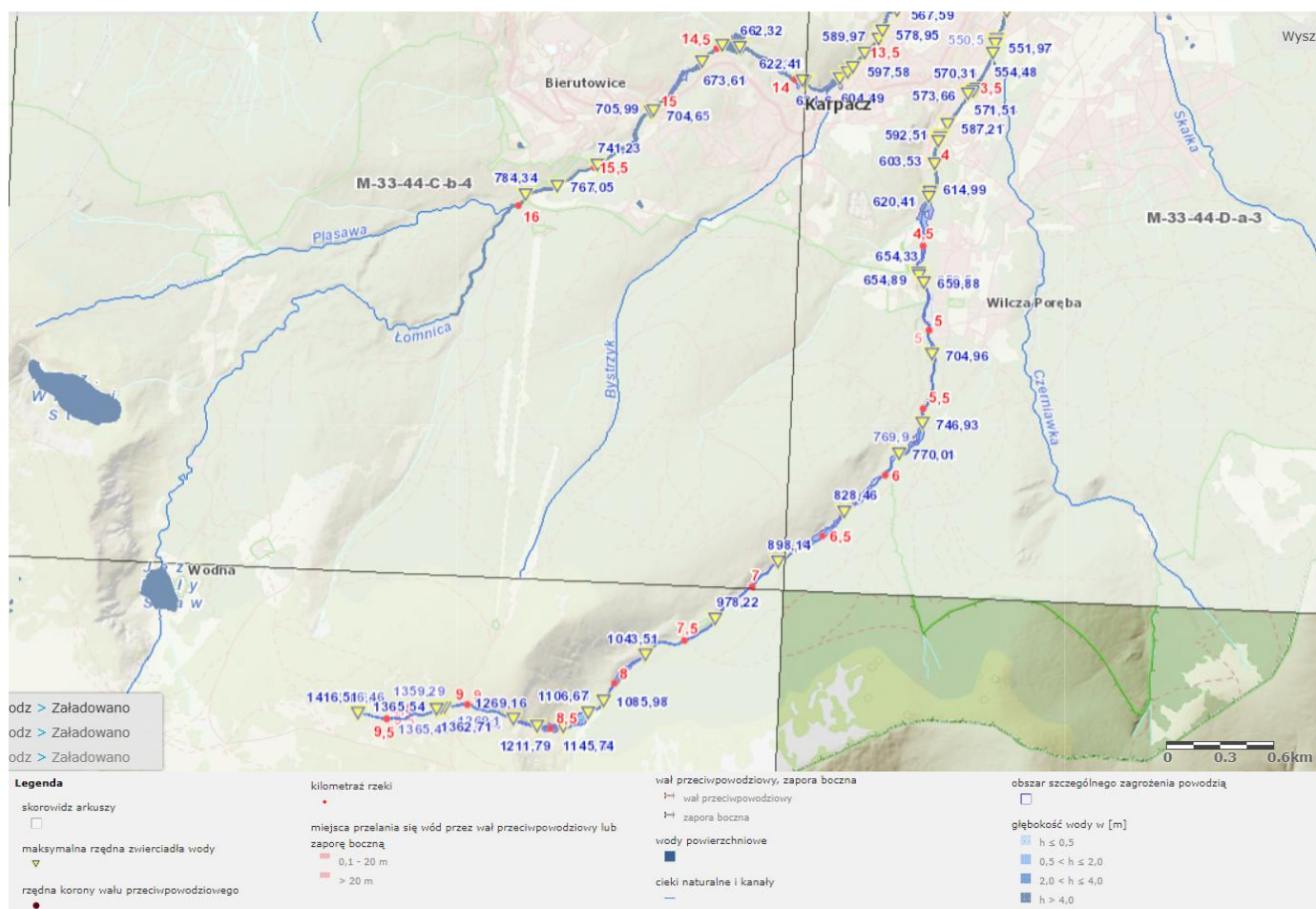
Rysunek 13 Mapy zagrożenia powodziowego dla gminy Karpacz z uwzględnieniem Q0,2%, Q1% oraz Q10% Źródło: Hydroportal Państwowego Gospodarstwa Wodnego Wody Polskie wody.isok.gov.pl . [dostęp: 16.04.2025].
